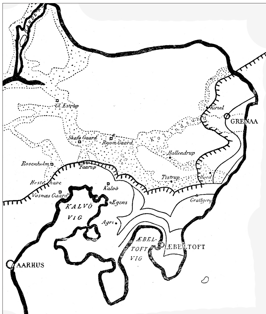
Kort over isafsmeltingen i Djursland. De tykke linier med små streger angiver israndens yderste stilling. Linierne bagved antyder morænevolde, der til dels er skudt op under israndspartiet. De prikkede arealer er smeltvandssletter. Den yderste, meget tykke, sorte linie er den nuværende kyst. (D. G. U.)
