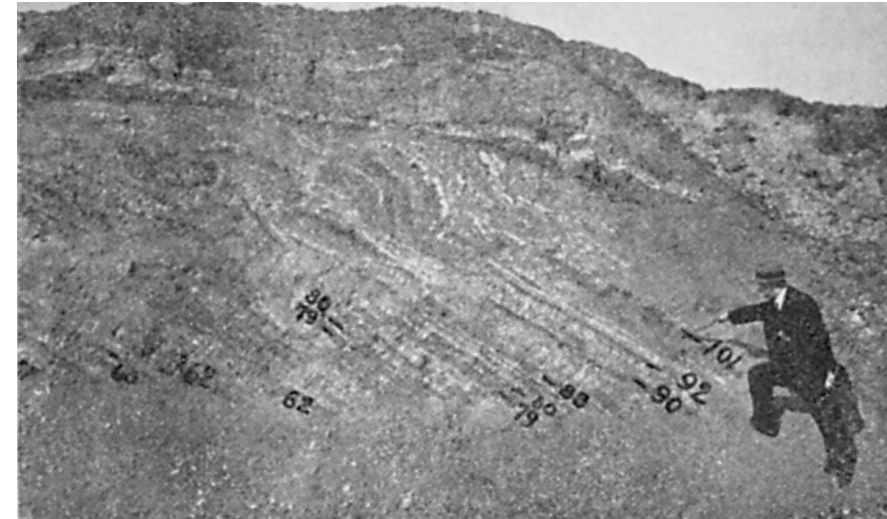
Parti fra klinten ved Ørby. Man ser her en hel række vulkanske askelag nummeret med tal. (D. G. U.)
