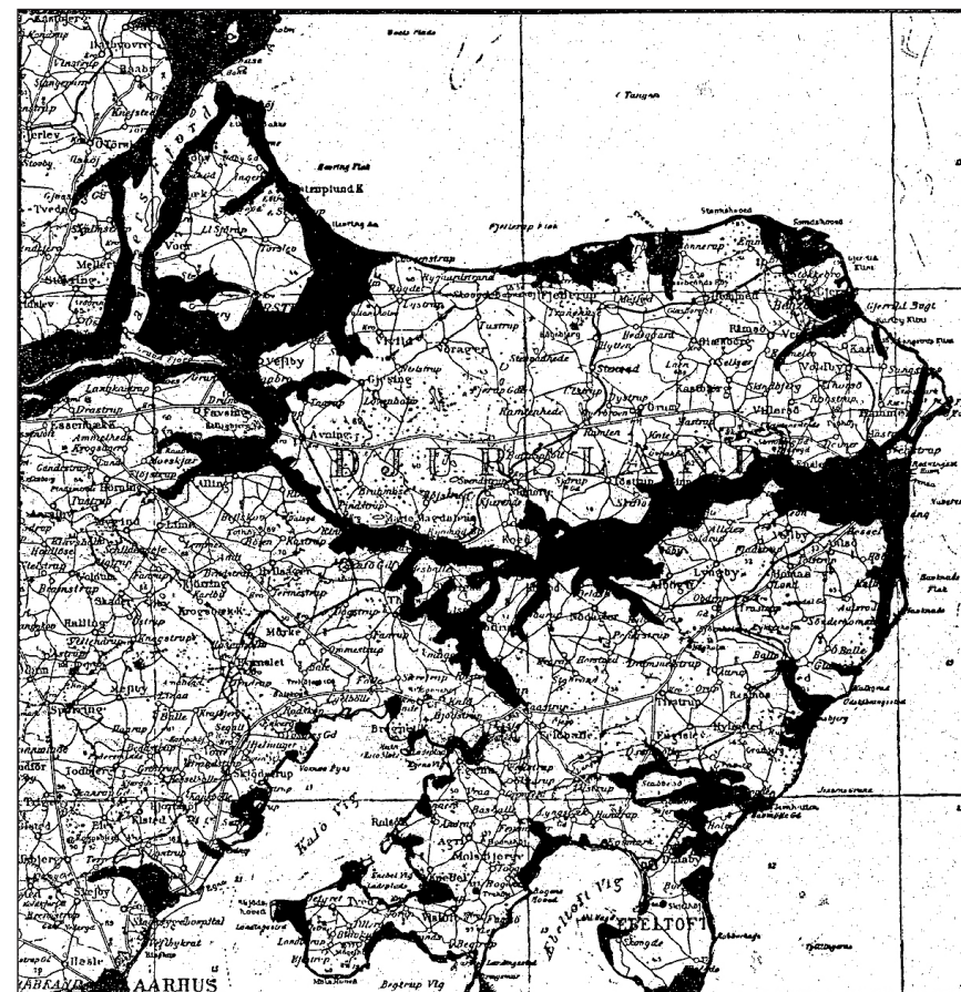
Kort over stenalderhavets udbredelse på Djursland. De med sort angivne partier er de dele af Djursland, der dengang, men ikke nu var dækket af havet. (Tegnet på grundlag af D. G. U. Kort).
